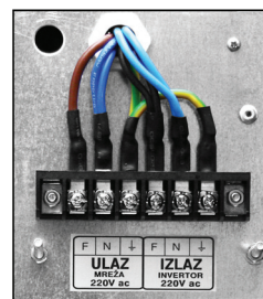
Izgled priključne kutije sa rasporedom klema
